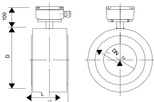
Rys.1a Wymiary czujników typu UC-057
