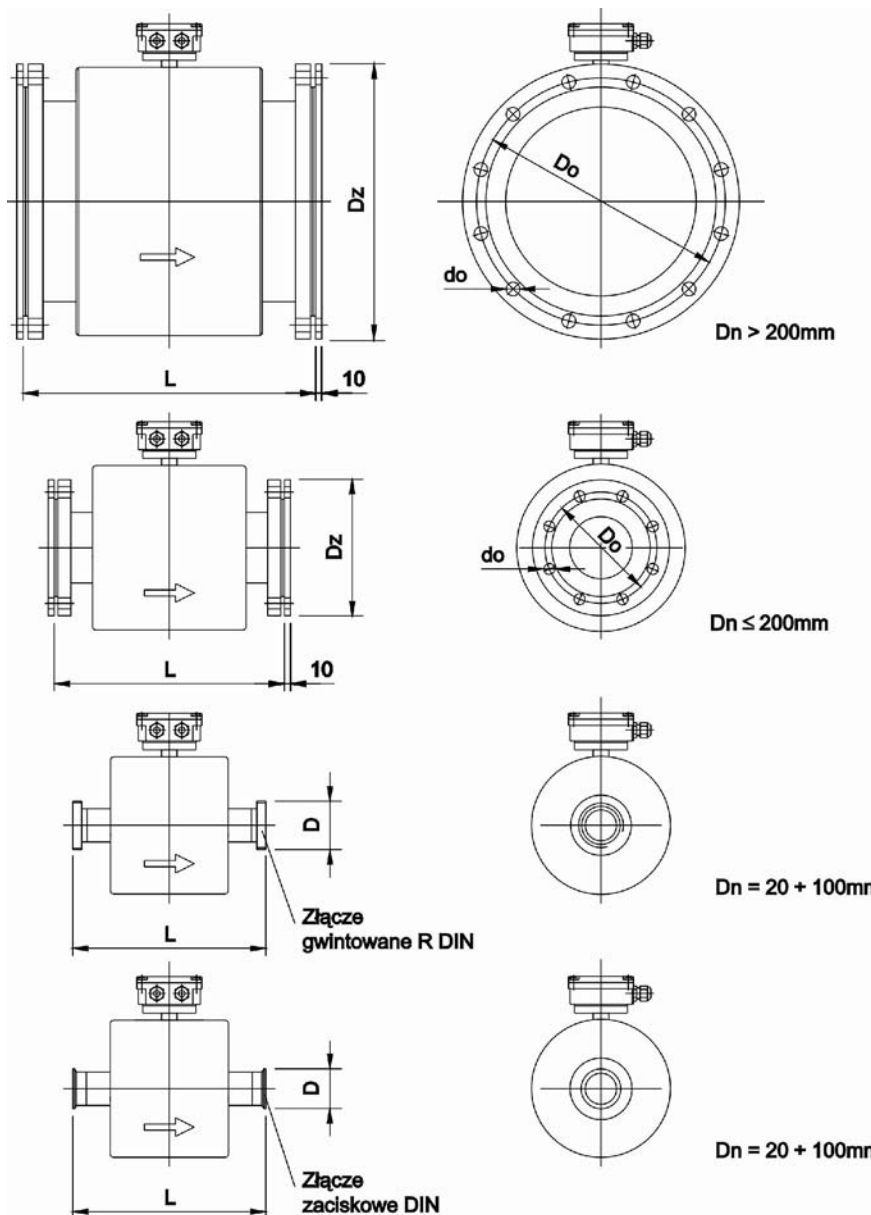
Rys.1 Wymiary czujników
