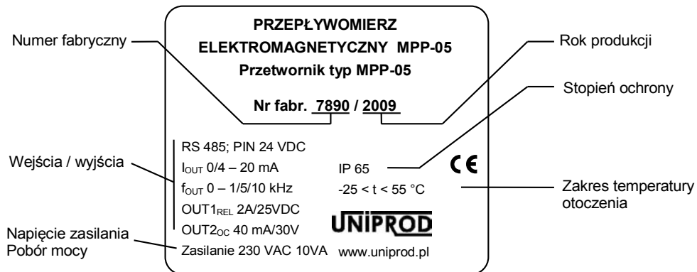
Tabliczka znamionowa czujnika
