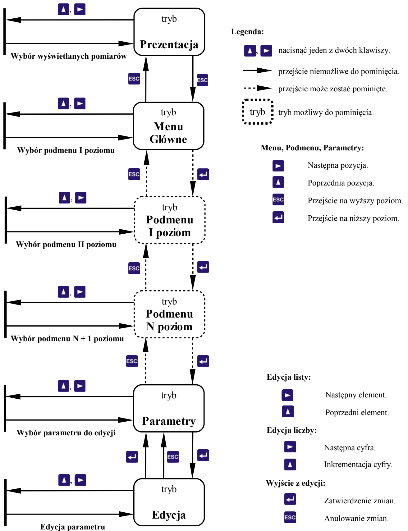
Uproszczony graf przejść między trybami pracy systemu menu.
