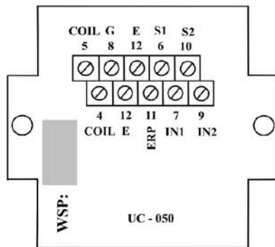
Płytkę połączeniową czujnika.
